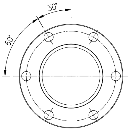
Ansicht (View) FL1+2
