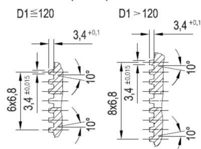
Ansicht (View) X
